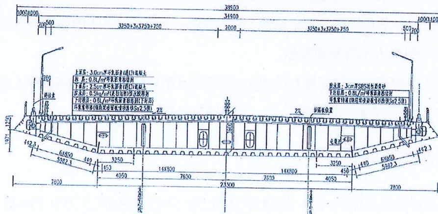
图 1-1 九江长江公路大桥主桥钢桥面横断面图
